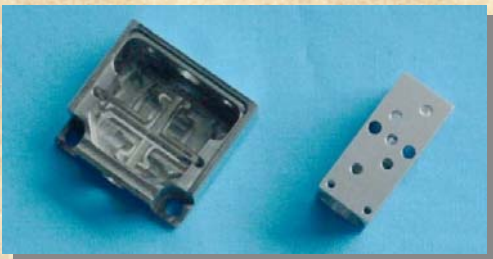
SUS304 コネクターボックス
