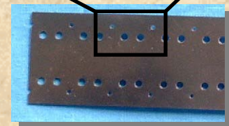
SUS303 t=0.2にφ0.2の 穴を空ける
