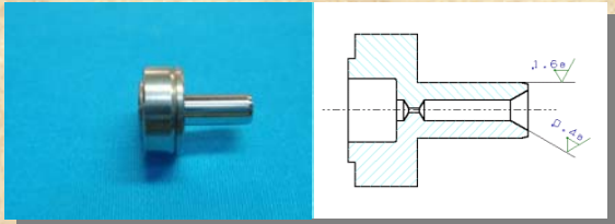
SUM24L 焼き入れ後Ra0.4・Ra1.6に加工 かつ、Ra0.4部を真円度0.3μmに切削加工
